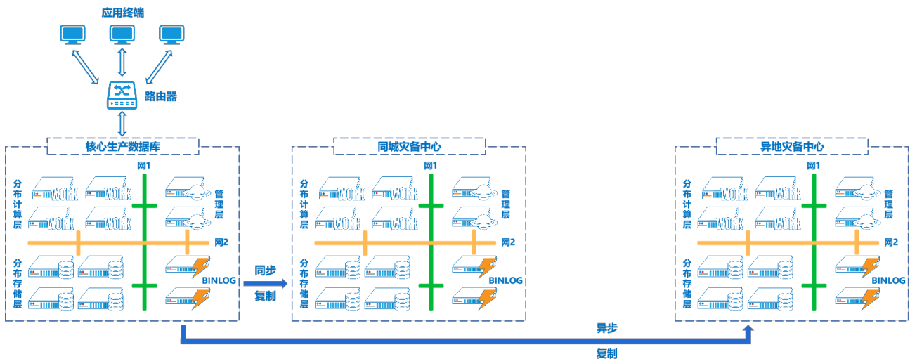
图 1-3 两地三中心
